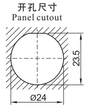
开孔尺寸 Panel cutout
